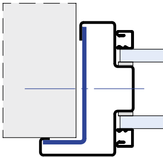
als Eckzarge mit L-Anker für Dübelmontage
