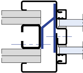
als 2-teilige Zarge auf Gipswand mit Z-Anker
