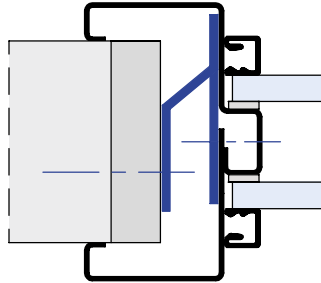
als 2-teilige Zarge auf Holzblindrahmen mit Z-Anker
