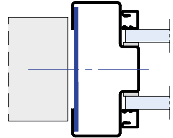
als 1-teilige Zarge in Wandlaibung mit Flachanker
