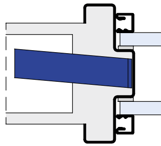
als Mauerwerkzarge (Eingießzarge) mit Maueranker
