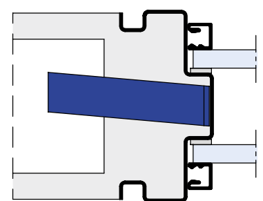
als Mauerwerkzarge (Eingießzarge) mit Schattennut, Befestigung Maueranker
