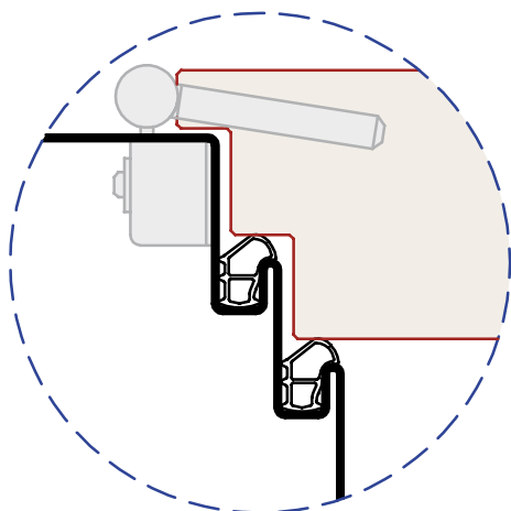
doppelt gefälztes Türblatt
