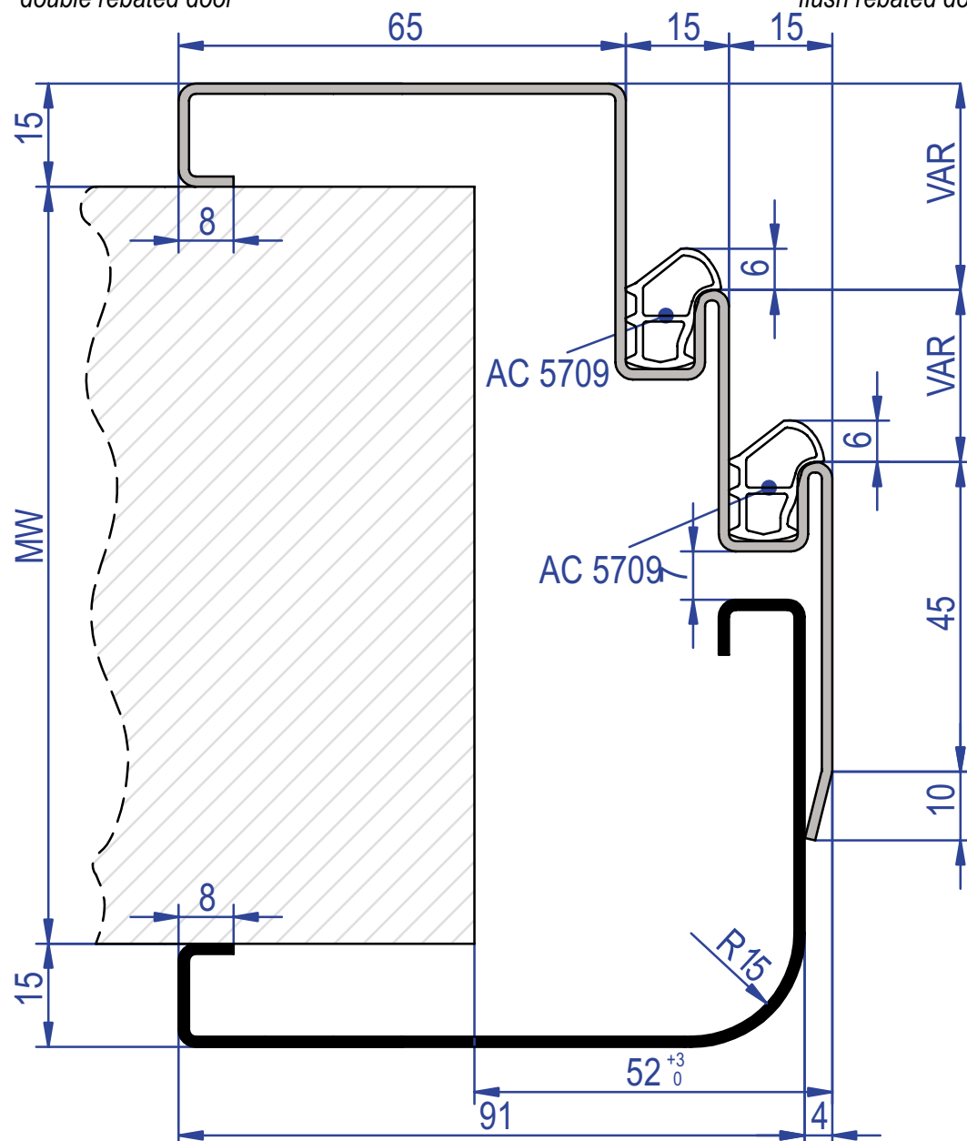
doppelt gefälztes Türblatt porta a doppia battuta double rebated door
