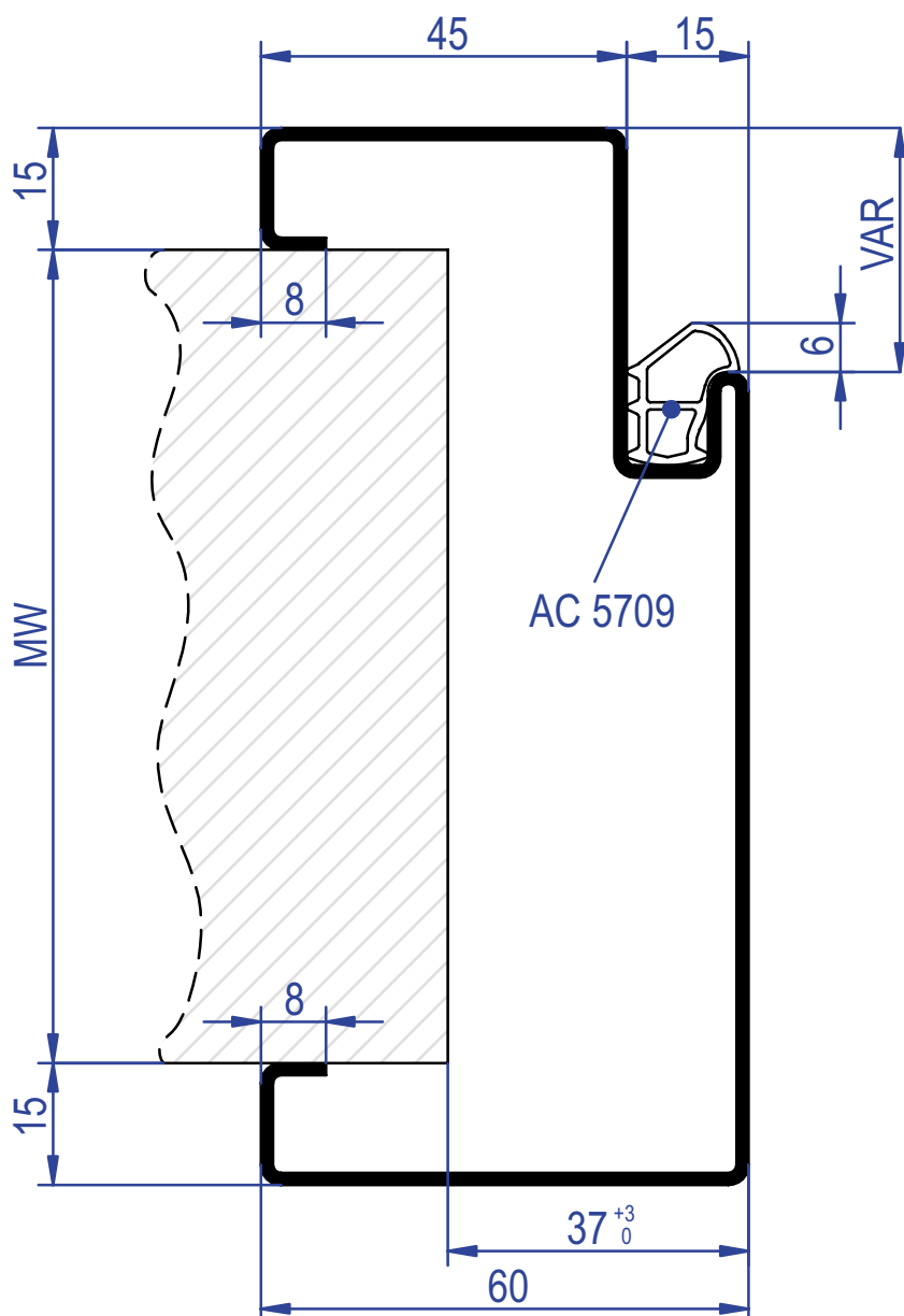
gefälztes Türblatt porta con battuta rebated door
