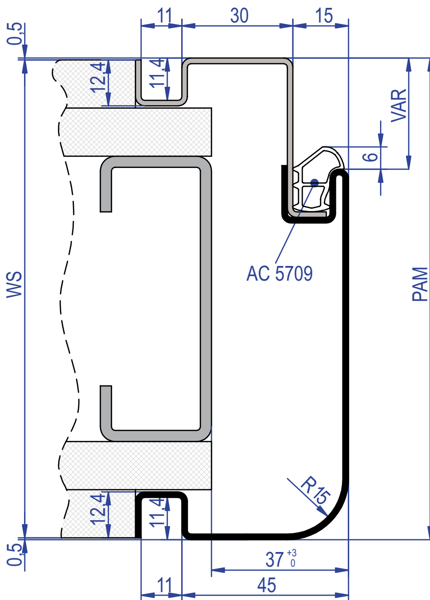
gefälztes Türblatt porta con battuta rebated door
