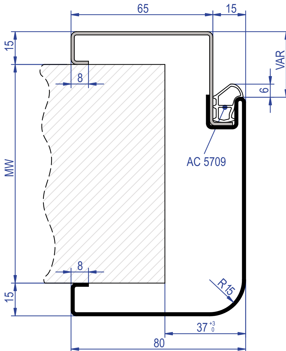
gefälztes Türblatt porta con battuta rebated door
