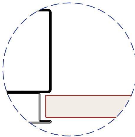
Stahlzargen für Schiebetüren casseperte per porte scorrevoli steel frames for sliding doors
