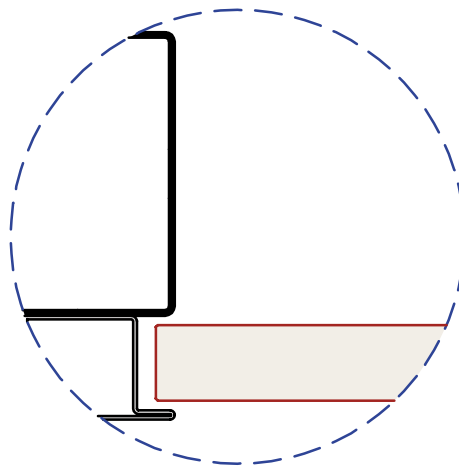
Stahlzargen für Schiebetüren casceporte per porte scorrevoli steel frames for sliding doors
