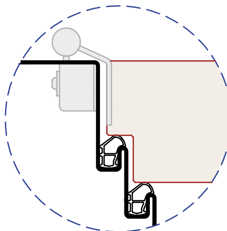
stumpf gefälztes Türblatt
