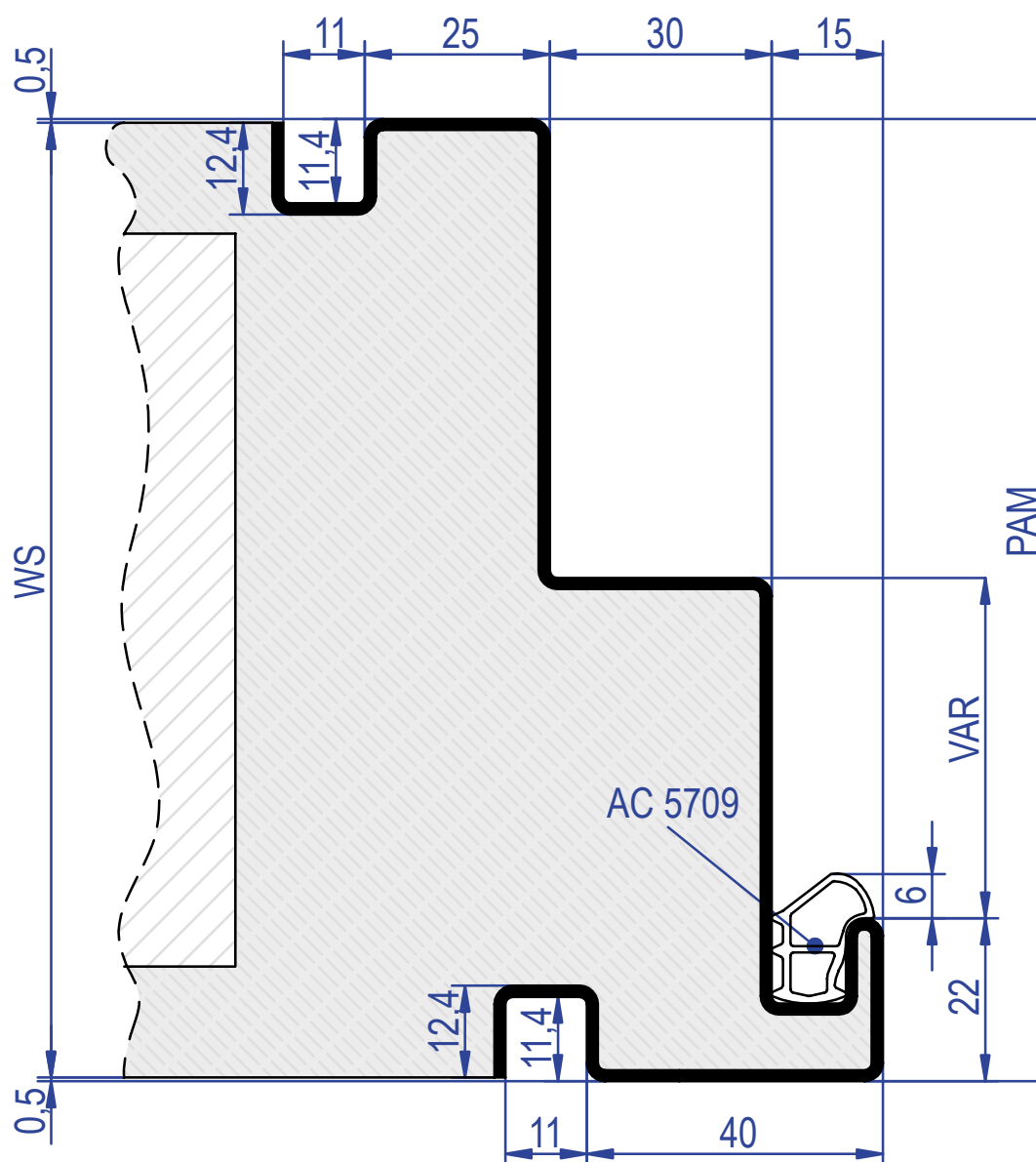
doppelt gefälztes Türblatt porta a doppia battuta double rebated door
