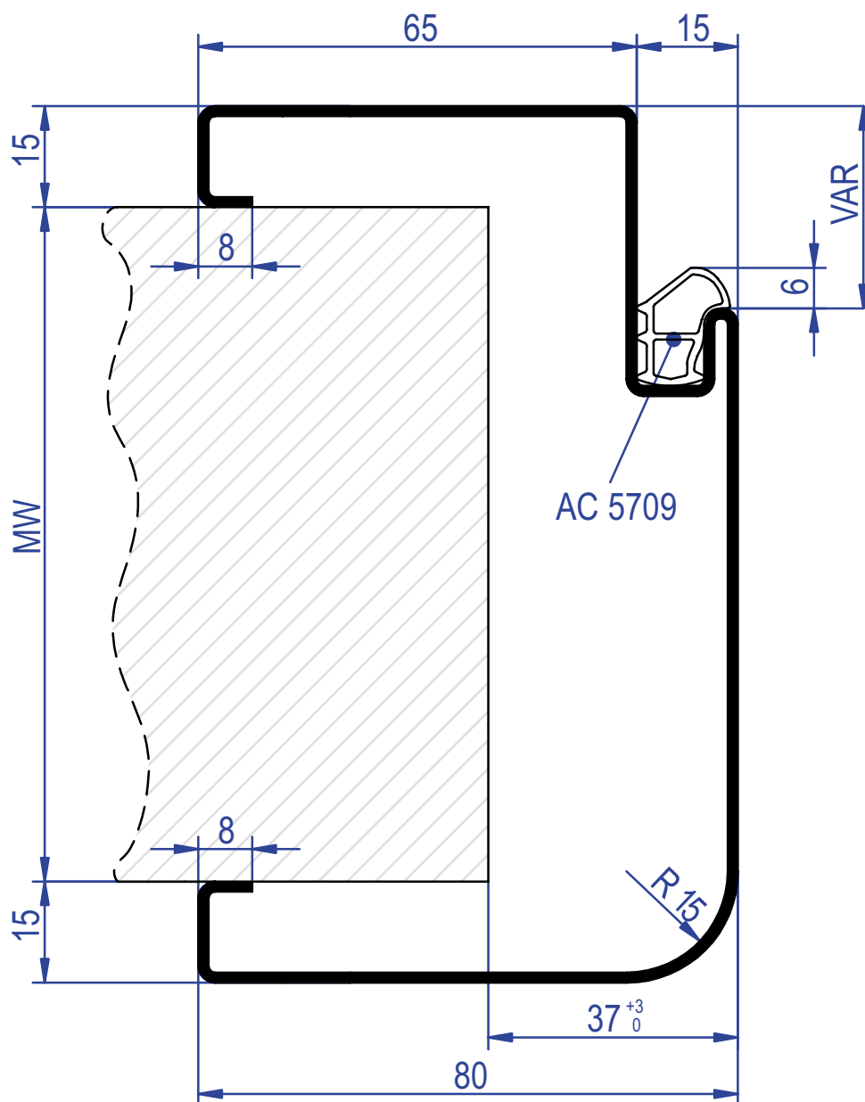
gefälztes Türblatt porta con battuta rebated door
