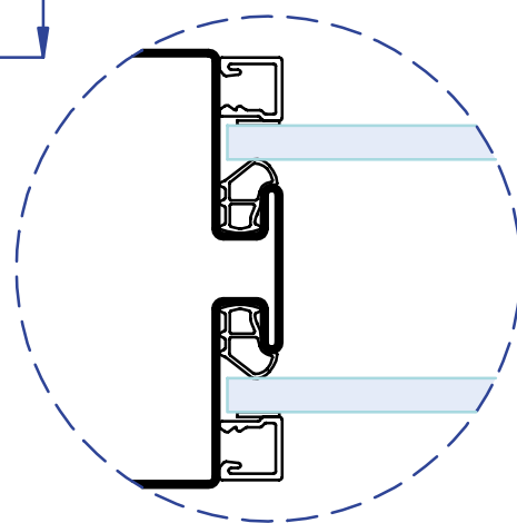
doppelt verglastes Fenster finestra con doppia vetrata window with 2 glasses
