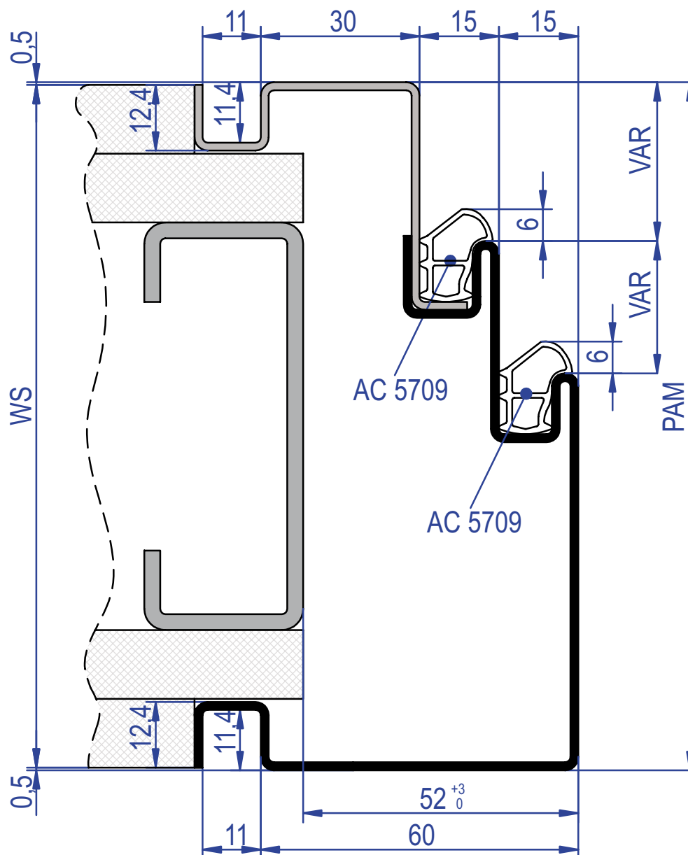
doppelt gefälztes Türblatt porta a doppia battuta double rebated door
