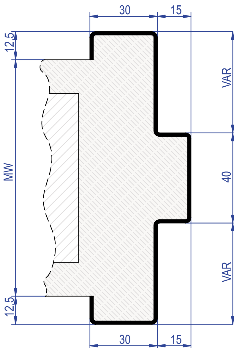
doppelt verglastes Fenster finestra con doppia vetrata window with 2 glasses
