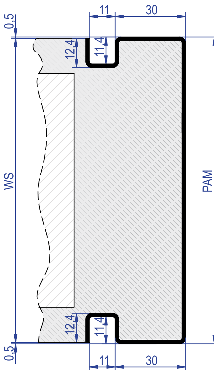
Durchgangszargen telai di passaggio trespassing frames
