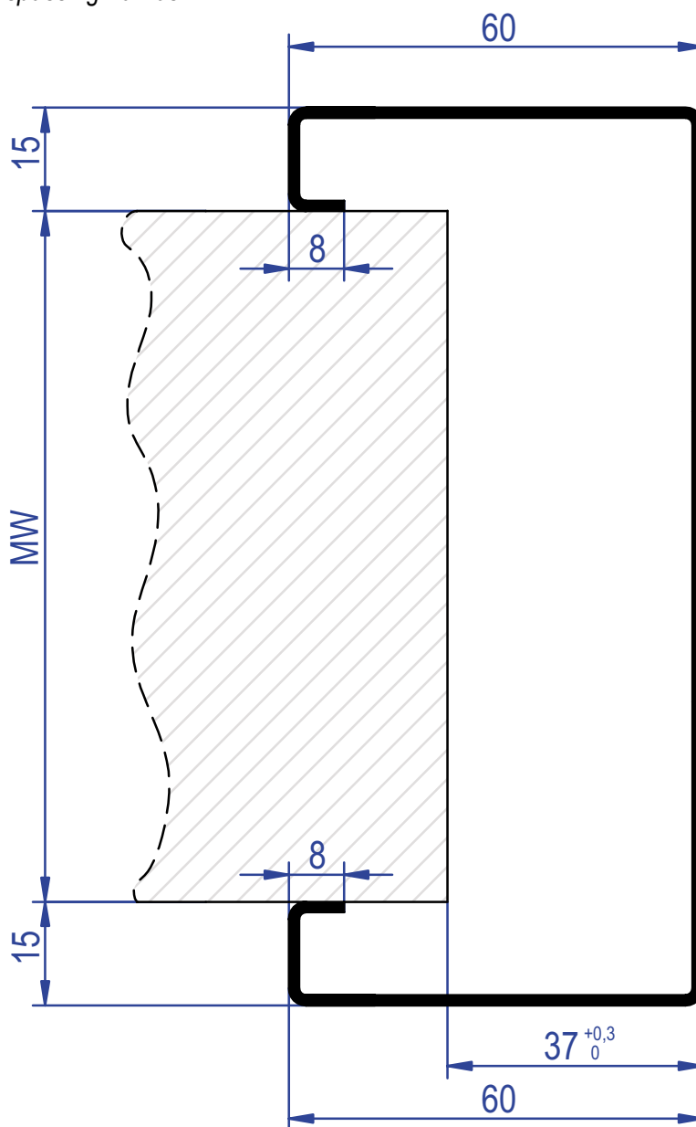
Durchgangszargen telai di passaggio trespassing frames
