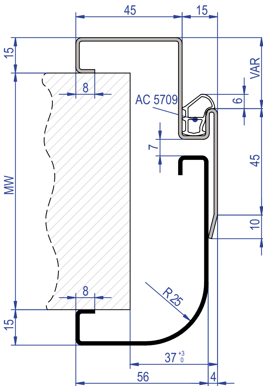
gefälztes Türblatt porta con battuta rebated door
