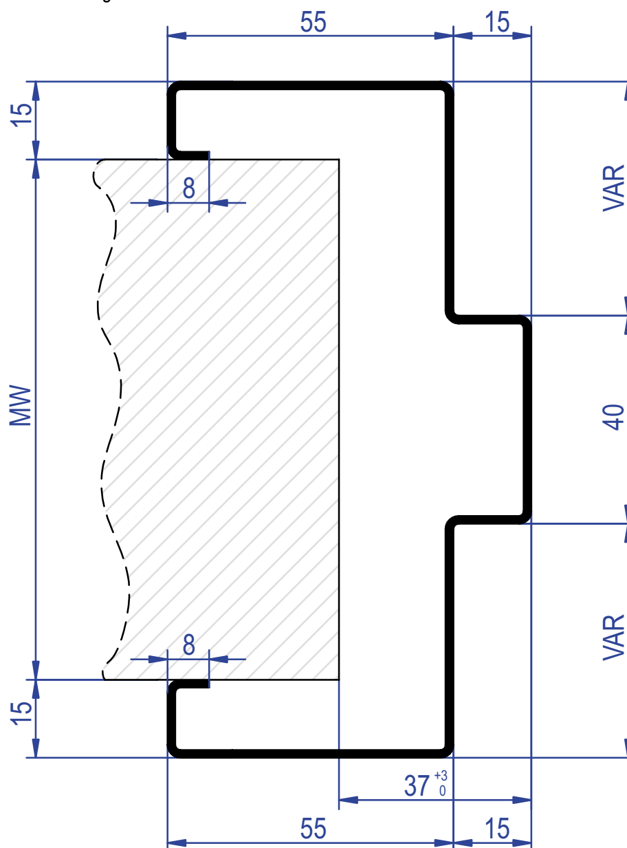
doppelt verglastes Fenster finestra con doppia vetrata window with 2 glasses
