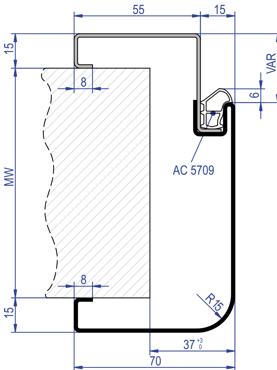
gefälztes Türblatt porta con battuta rebated door
