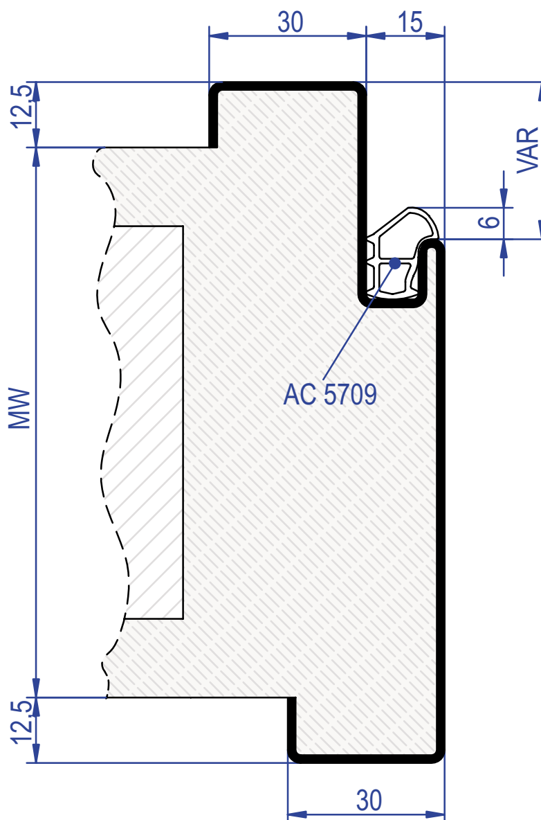
gefälztes Türblatt porta con battuta rebated door
